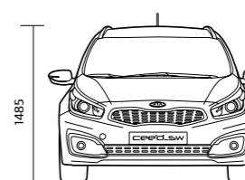
cee'd Sportswagon: dimensões exteriores (mm)
