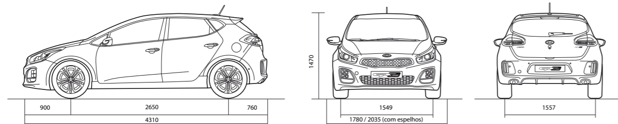
cee'd 5 portas GT Line: dimensões exteriores (mm)
