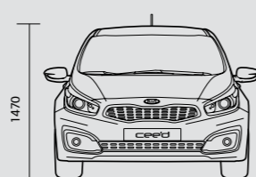
cee'd 5 portas: dimensões exteriores (mm)
