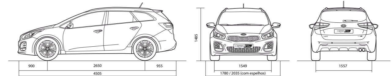
cee'd Sportswagon GT Line: dimensões exteriores (mm)
